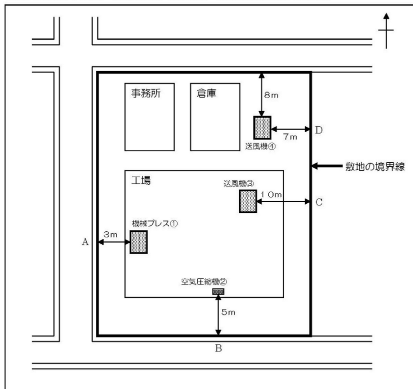
《例》敷地の平面図・建物の配置状況図・特定施設の配置状況図
