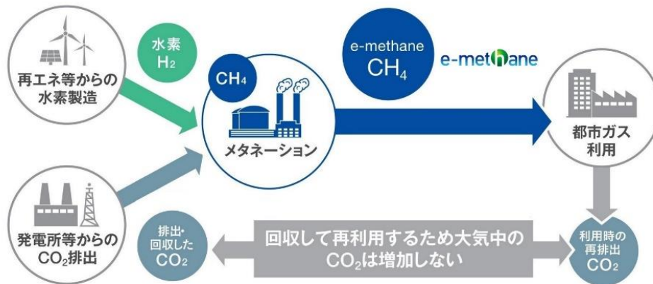
メタネーション概要 (出典：東京ガスホームページ)
